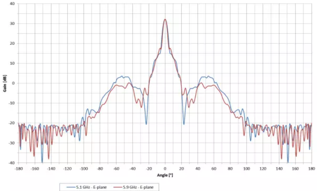
JRC-32DD Duplex Precision - E-plane
