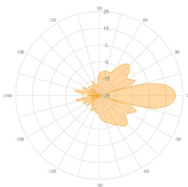
N5-X20 (20 dBi)
