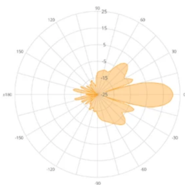
N5-X20 (20 dBi)
