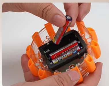
Montaż baterii
