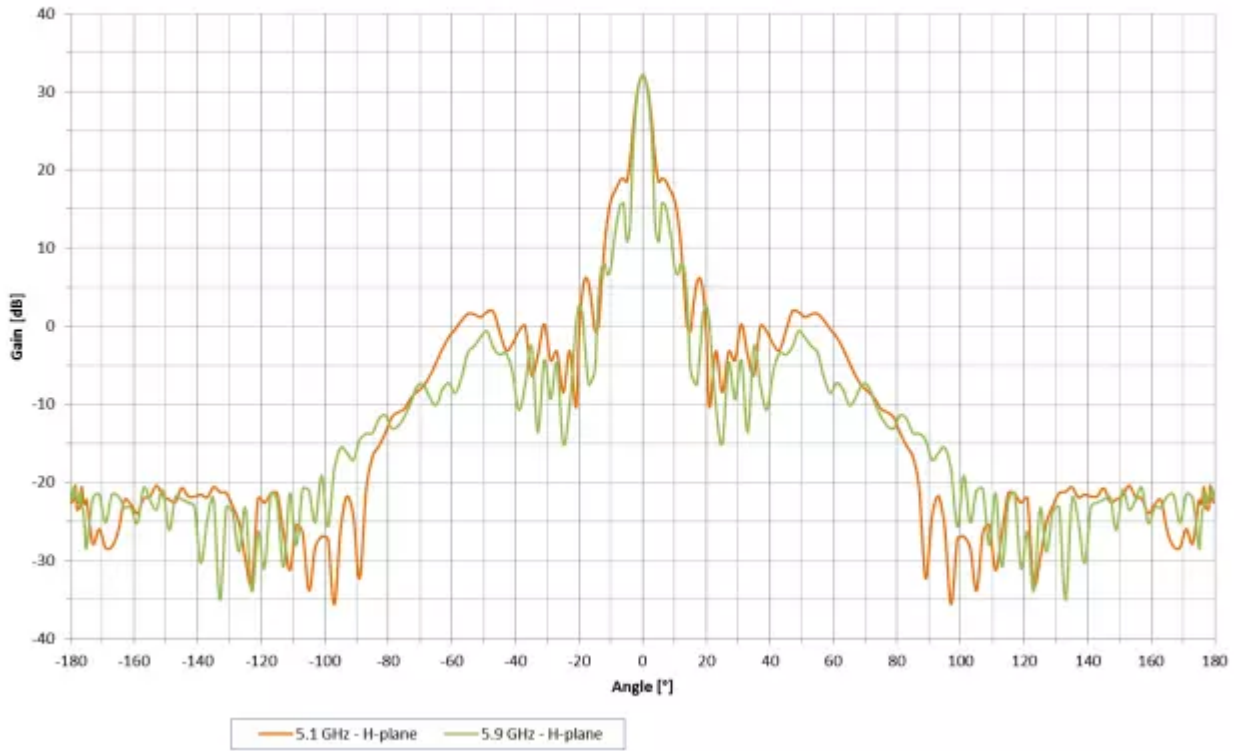
JRC-32DD DupLEX Precision - H-plane
